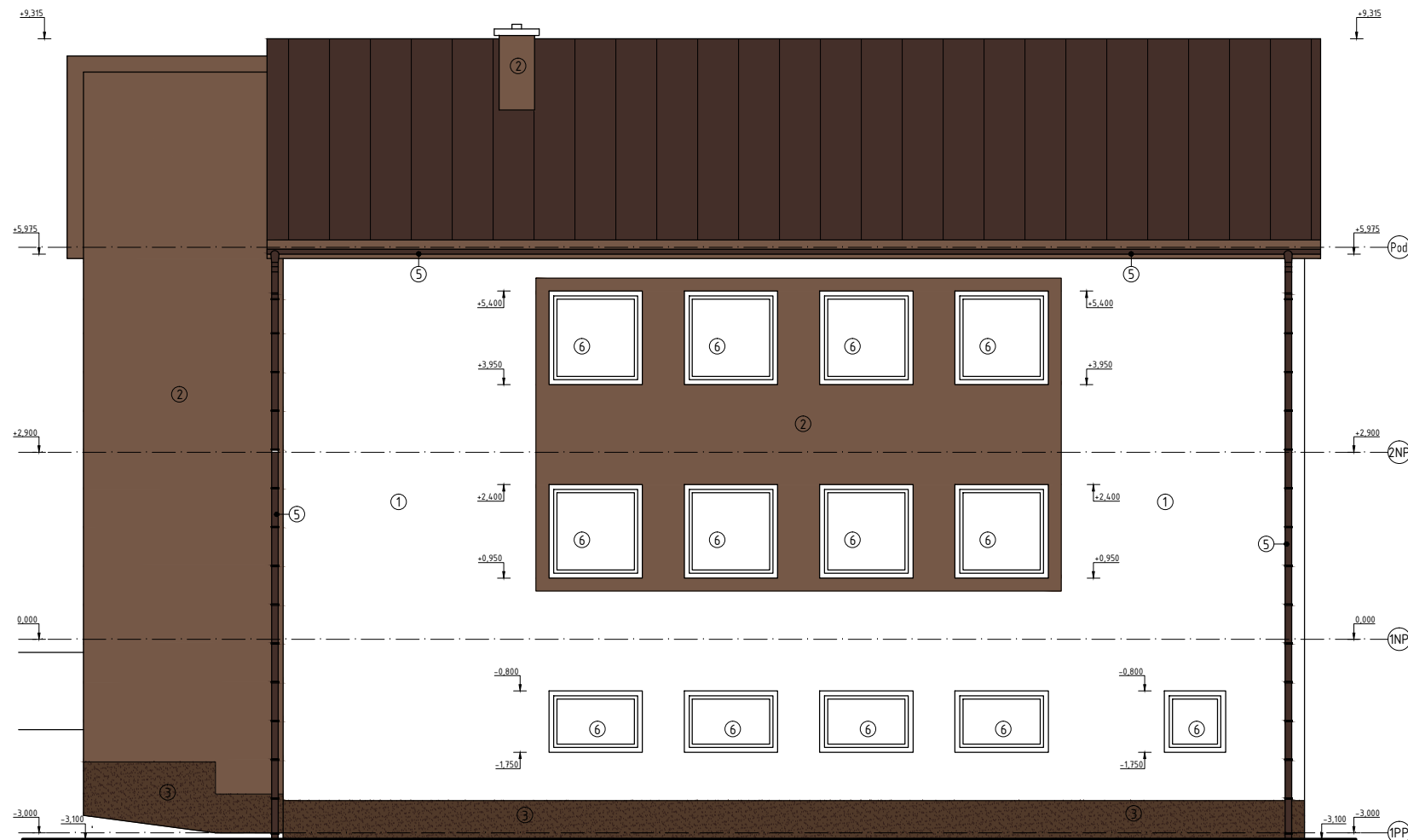
POHĽAD SEVEROVÝCHODNÝ
